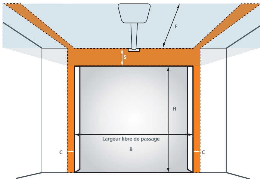
B = Largeur, H = Hauteur, C = Ecoïçon, S = Linteau, F = Profondeur
